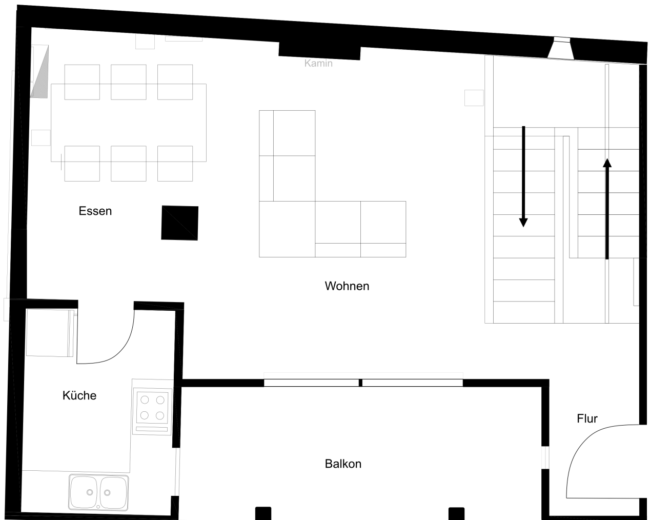
1. Obergeschoss
